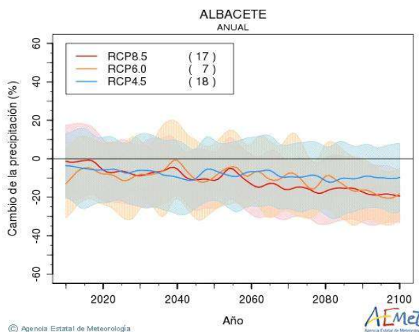
Imagen 15 – Gráfico de predicción del cambio de la precipitación. Fuente: AEMET
