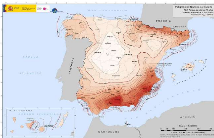
Imagen 12 – Mapa de peligrosidad sísmica de España 2015 (en valores de aceleración). Fuente: IGN.
