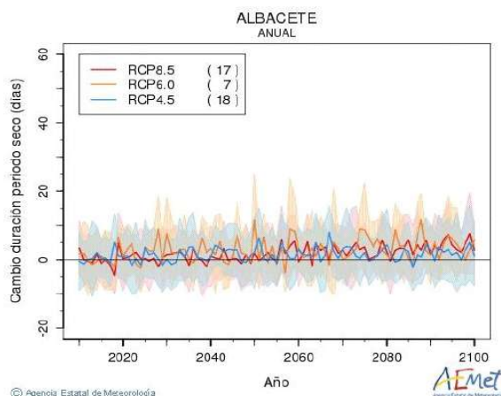
Imagen 18 – Gráfico de predicción del cambio de la duración del periodo seco. Fuente: AEMET
