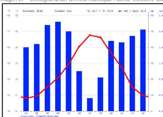
Imagen 07 – Climograma del término municipal. Fuente: CLIMATE-DATA
